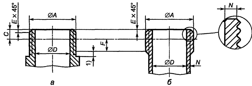
Рисунок 3 — Наружное коническое резьбовое соединение с резьбой по ГОСТ 6211
