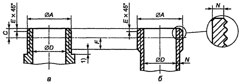
Рисунок 4 — Наружное модифицированное коническое резьбовое соединение Rk по ГОСТ 6211
