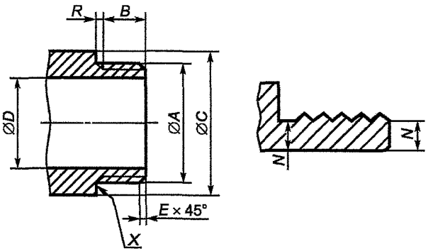
Рисунок 5 — Наружное цилиндрическое резьбовое соединение по ГОСТ 6357
